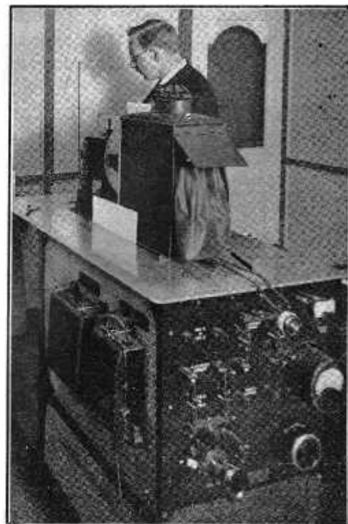
De Baird televisie-zender compleet
