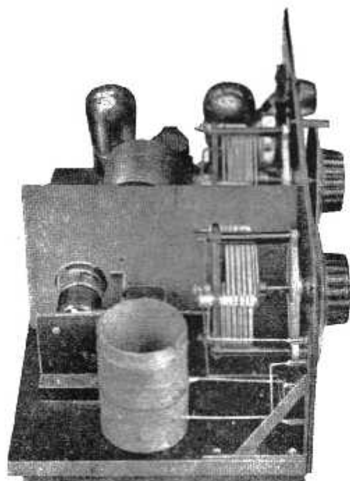
Het hoogfrequent-gedeelte
